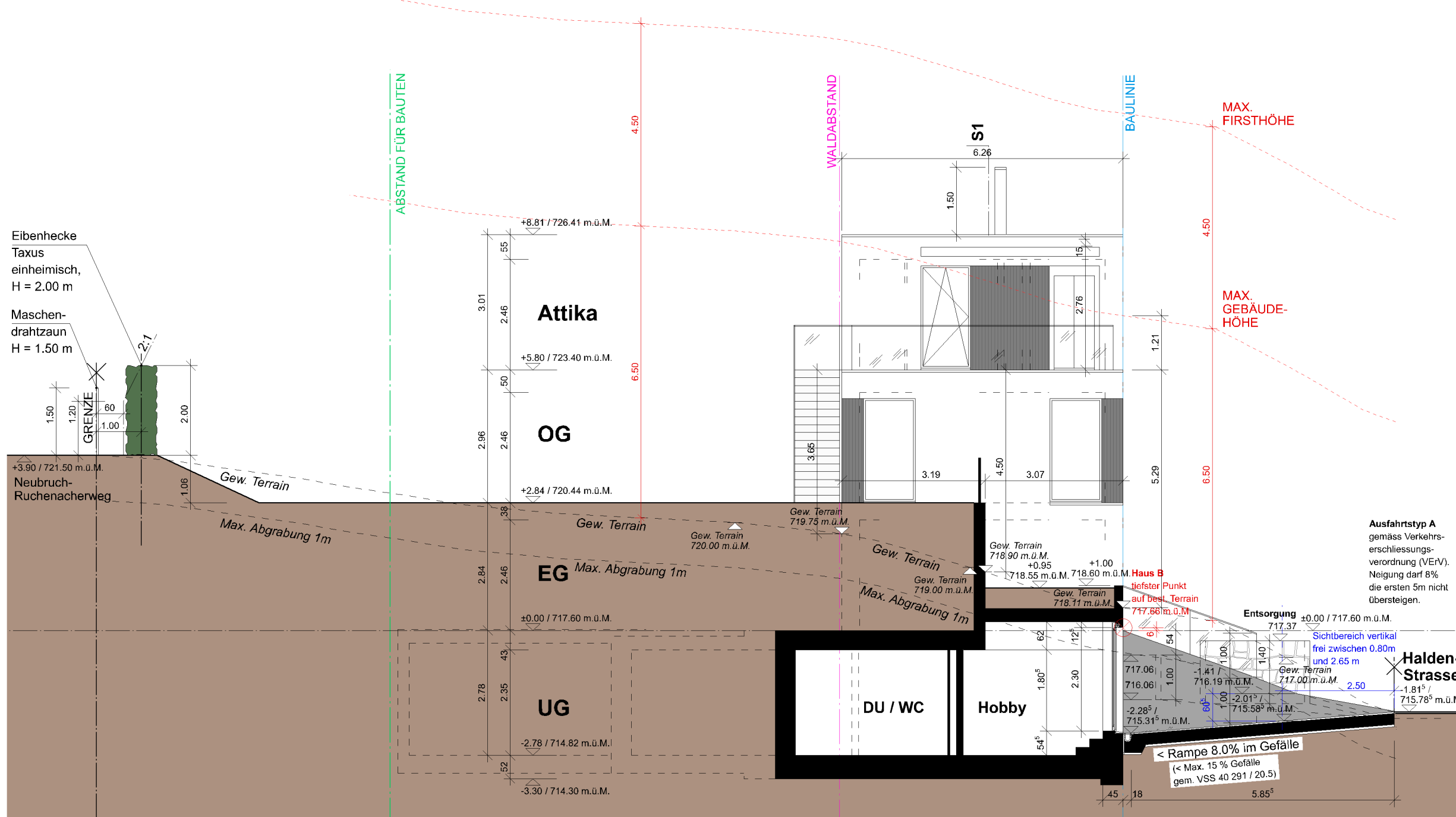
Westfassade Haus B
