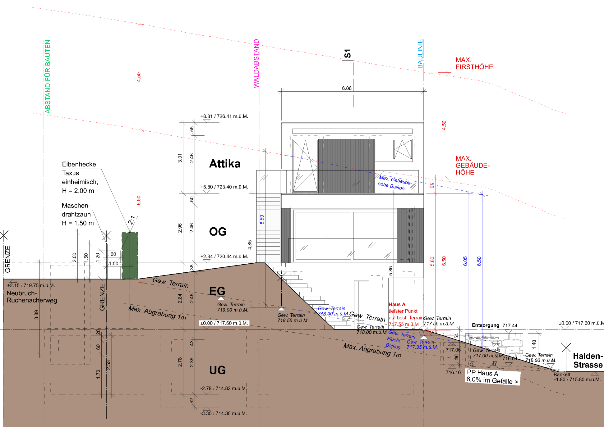
Westfassade Haus A
