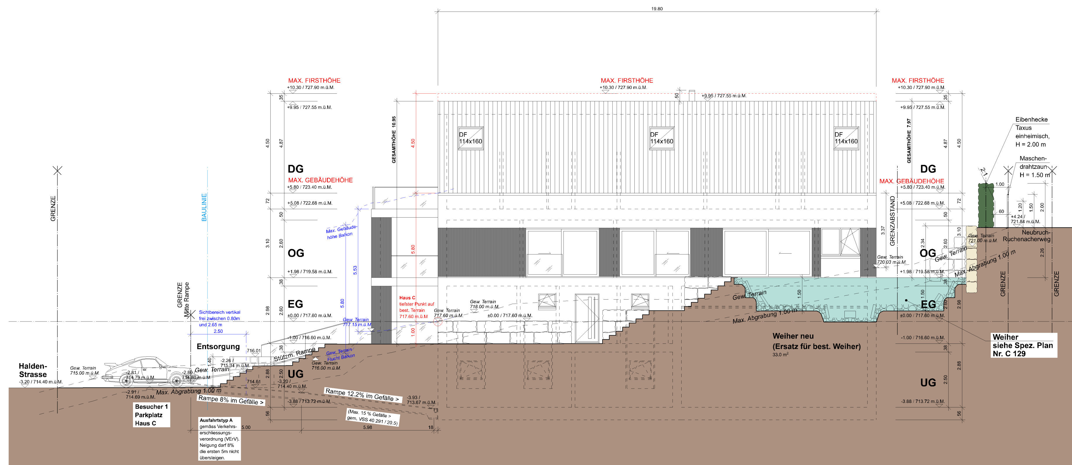
Ostfassade Haus C
