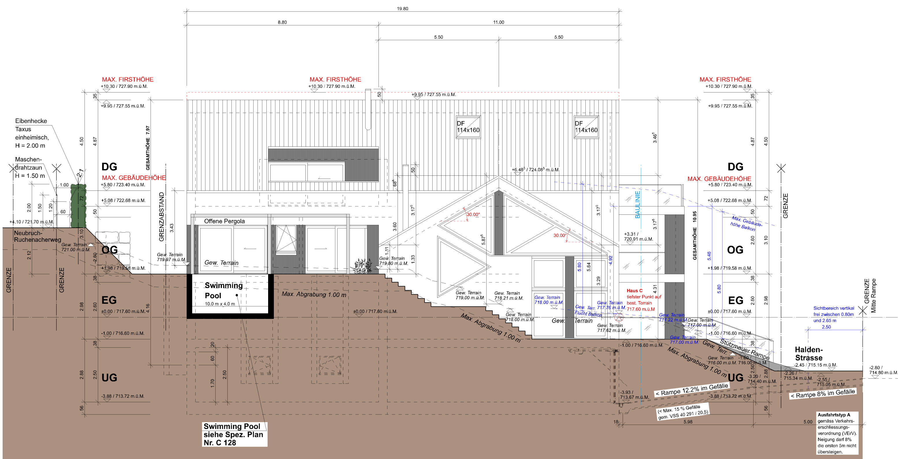
Westfassade Haus C
